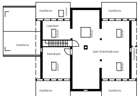
Dachgeschoss
