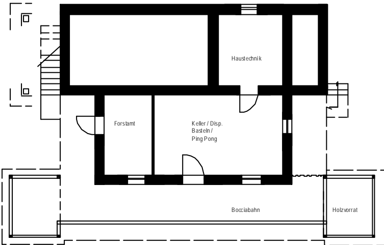
Kellergeschoss
