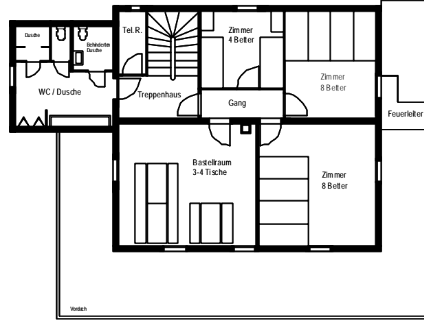
1 Obergeschoss
