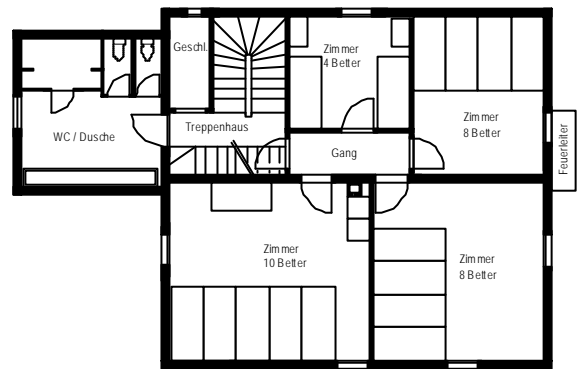
2 Obergeschoss
